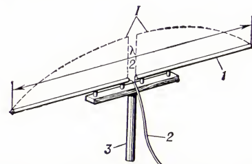
Простая телевизионная антенна: 1 — полуволновой вибратор; 2 — фидер; 3 — подставка. Пунктиром показано распределение тока I вдоль вибратора; λ — длина рабочей волны.
